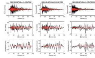
Şekil E. 3-12. Kayın-1 için ivme, hız ve deplasman zaman serileri (2475 yıl).
